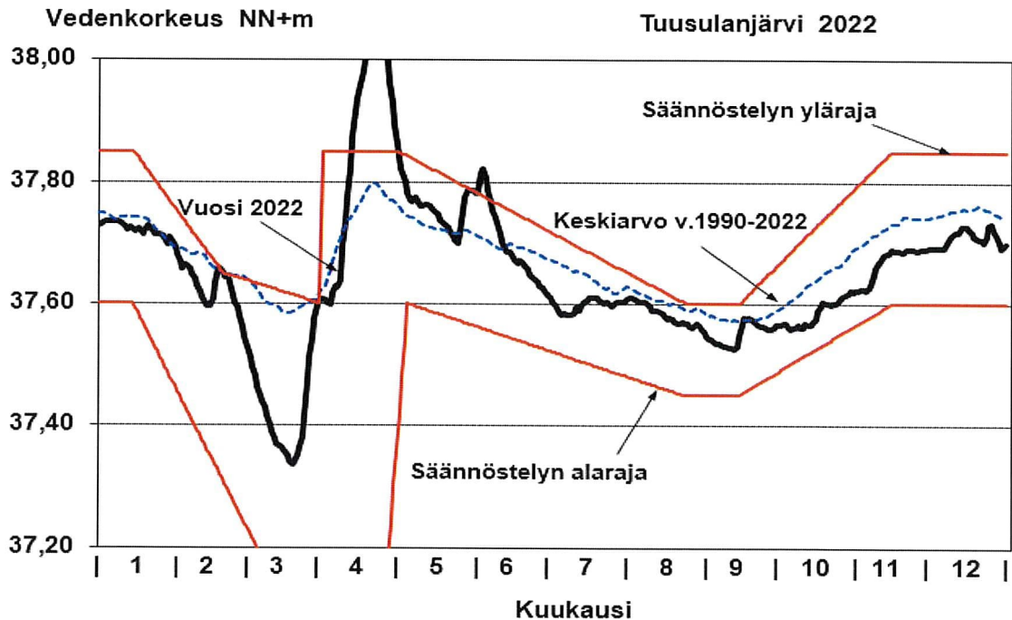
Kuva 1 Tuusulanjärven vedenkorkeus suhteessa säännöstelyrajoihin vuonna 2022.
